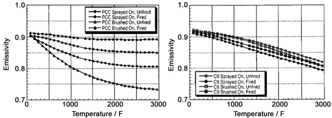
图 36 PCC 涂层和 C-9 涂层的辐射率随温度变化的关系 [313]
