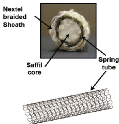
图 39 基线密封结构形式 Figure 39 Schematic of baseline seal structure
