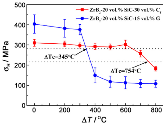
图 11 ZrB 2 -SiC-G 和 ZrB 2 -SiC-C f 复合材料的热冲击残余强度-热冲击温差曲线 [90]
