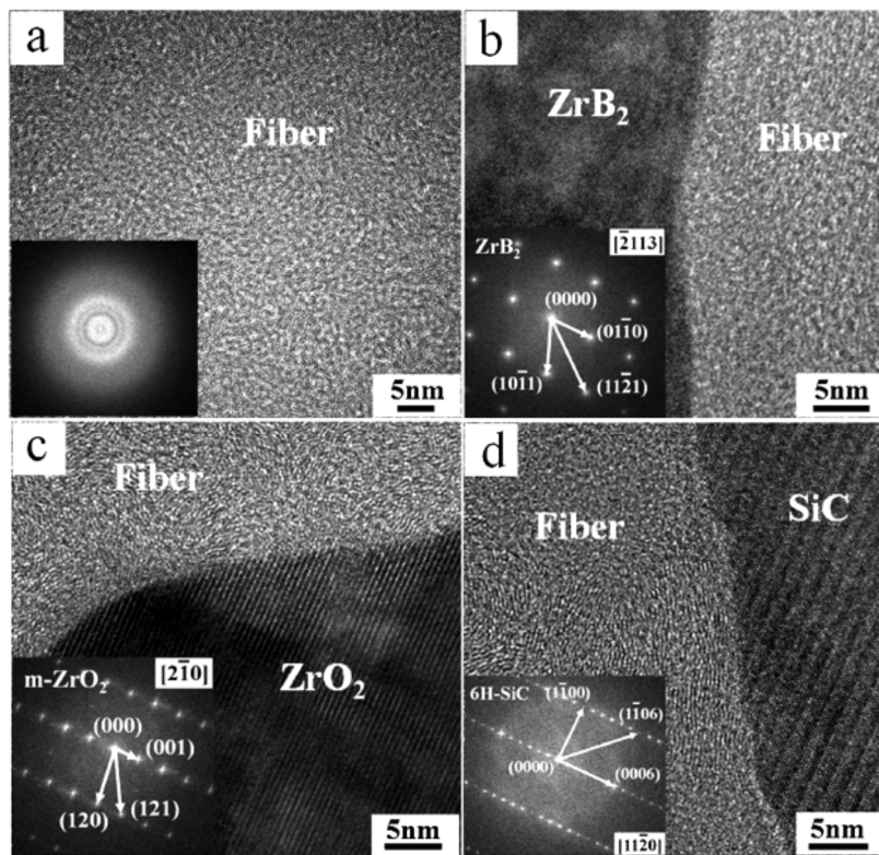
图 8 ZrB 2 -SiC-C f 复合材料中碳纤维与陶瓷基体的界面透射照片 [90]
