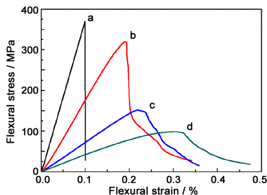
图 10 ZrB 2 -SiC-C f 复合材料的应力应变曲线 [90] Figure 10 Stress-strain curves of ZrB 2 -SiC-C f [90] (a) ZrB 2 -20vol%SiC-20vol%C f ; (b) ZrB 2 -20vol%SiC-30vol%C f ; (c) ZrB 2 -20vol%SiC-20vol%C f ; (d) ZrB 2 -20vol%SiC-20vol%C f
