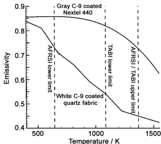
图 34 灰色 C-9 涂层和白色 C-9 涂层表面辐射率随温度的变化关系 [311]
