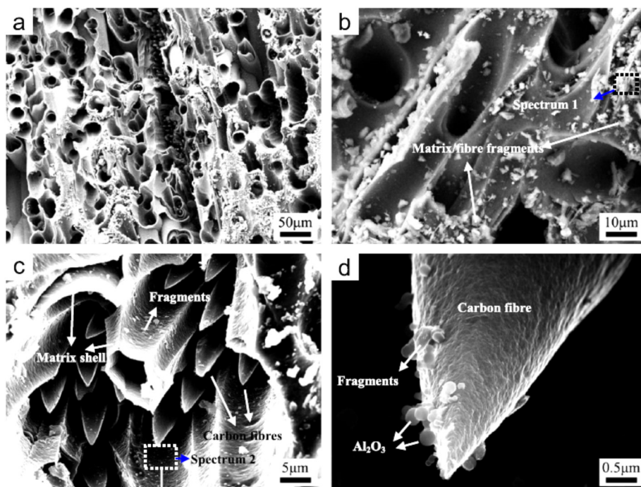
图 16 C/C-ZrC 复合材料喉衬发动机考核后的显微形貌 [173]
